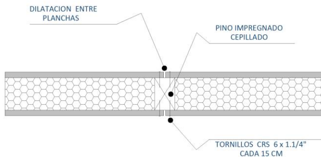
EMPALME PANELES MURO CON PIE DERECHO
